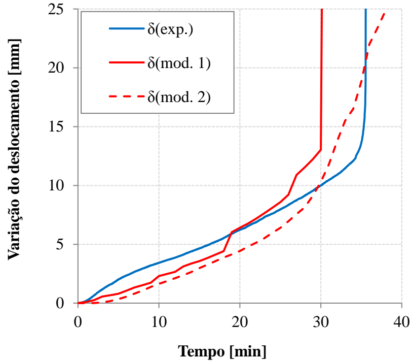
Figura 14. Resposta mecânica: resultados experimentais e analíticos para a viga NP-S1.
