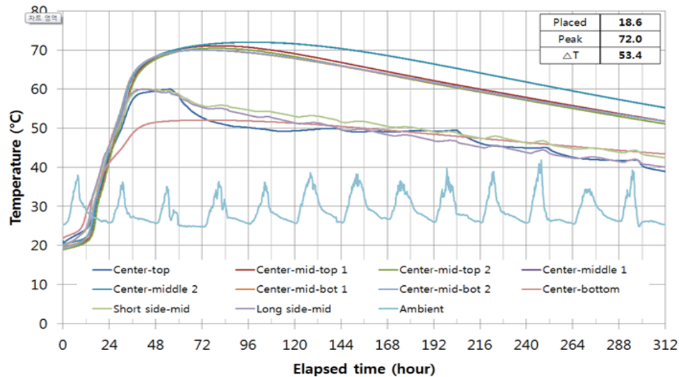
Figura 5. Resultado del monitoreo del aumento de temperatura del prototipo a escala real de la mega columna.
