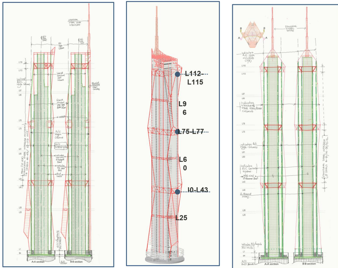
Figura 2a. Merdeka 118: Sistema estructural y sistema de estabilidad lateral Mega-Frame
