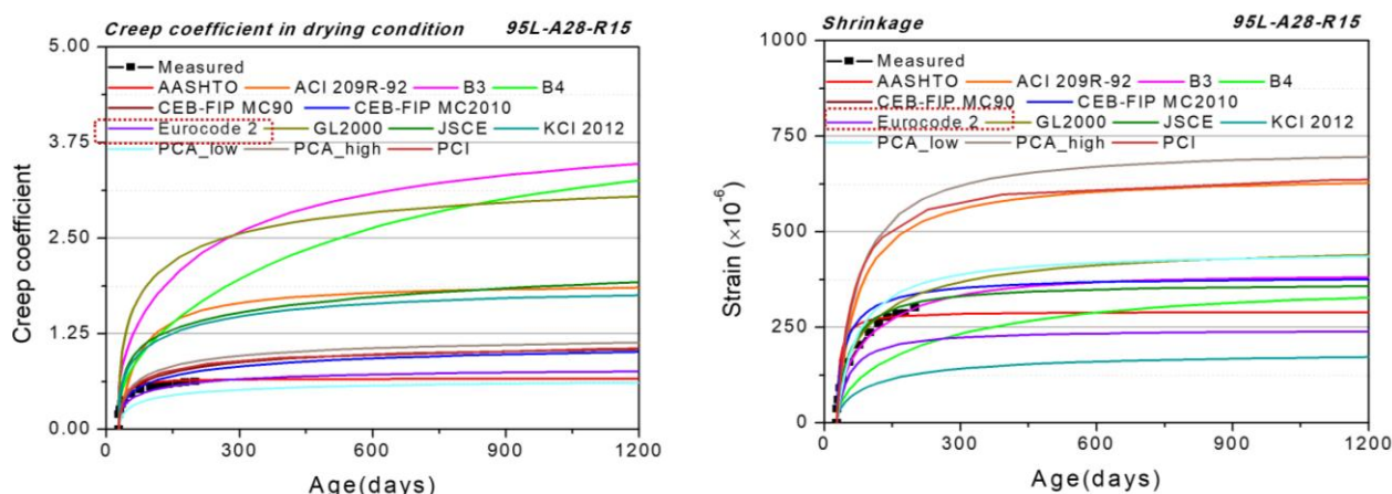
Figura 9. Pruebas de fluencia y contracción en tiempo real en un entorno totalmente controlado. Seúl, Corea.
