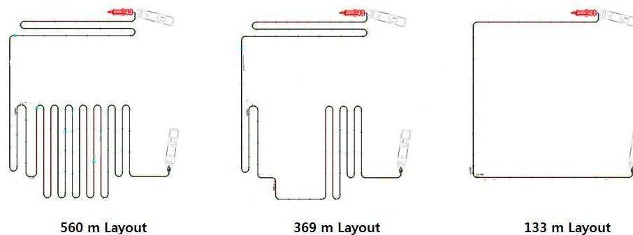
Figura 6. Diseño de tuberías y ubicación del sensor de presión.
