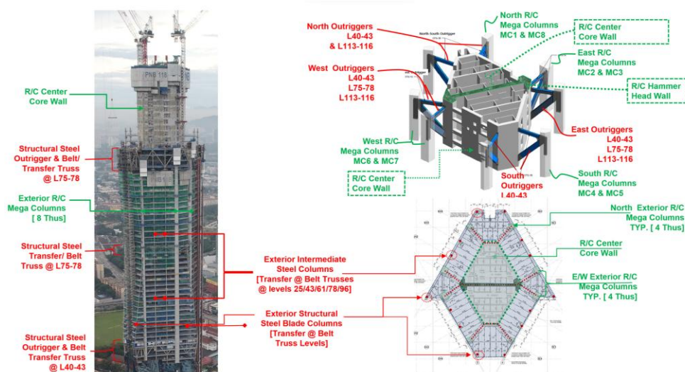
Figura 2b. Merdeka 118: Sistema estructural y sistema de estabilidad lateral Mega-Frame
