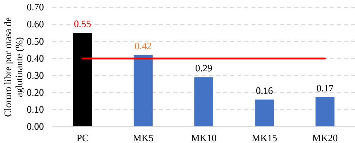
Figura 2. Porcentaje de cloruro libre en masa de aglutinante para el sistema con metacaolín, MK.
