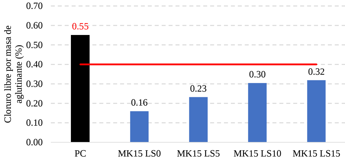
Figura 4. Porcentaje de cloruro libre en peso de aglutinante para el sistema metacaolín-calcáreo.
