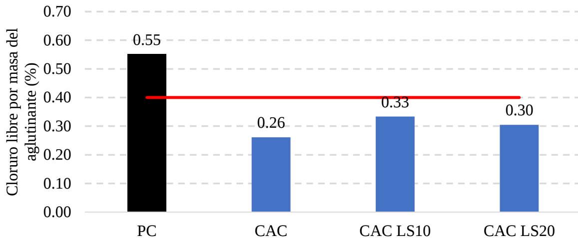
Figura 8. Porcentaje de cloruro libre por peso de ligante para el sistema CAC
