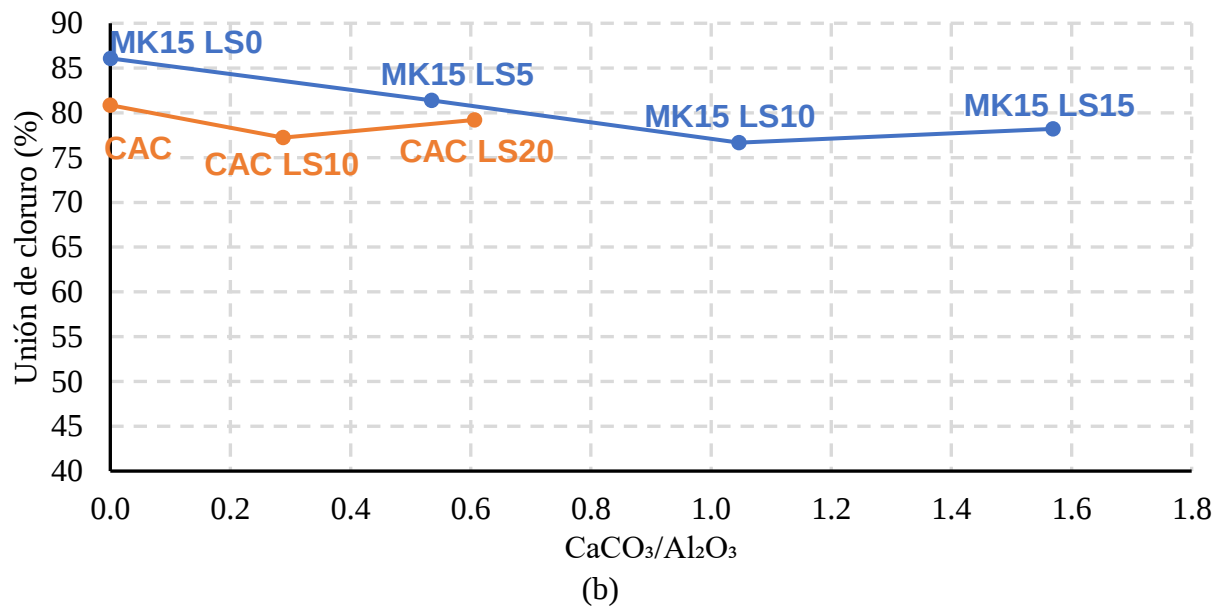
Figura 9. Capacidad de combinación de cloruro frente a a) razón \text{CaO}/\text{Al}_2\text{O}_3 y b) razón \text{CaCO}_3/\text{Al}_2\text{O}_3
