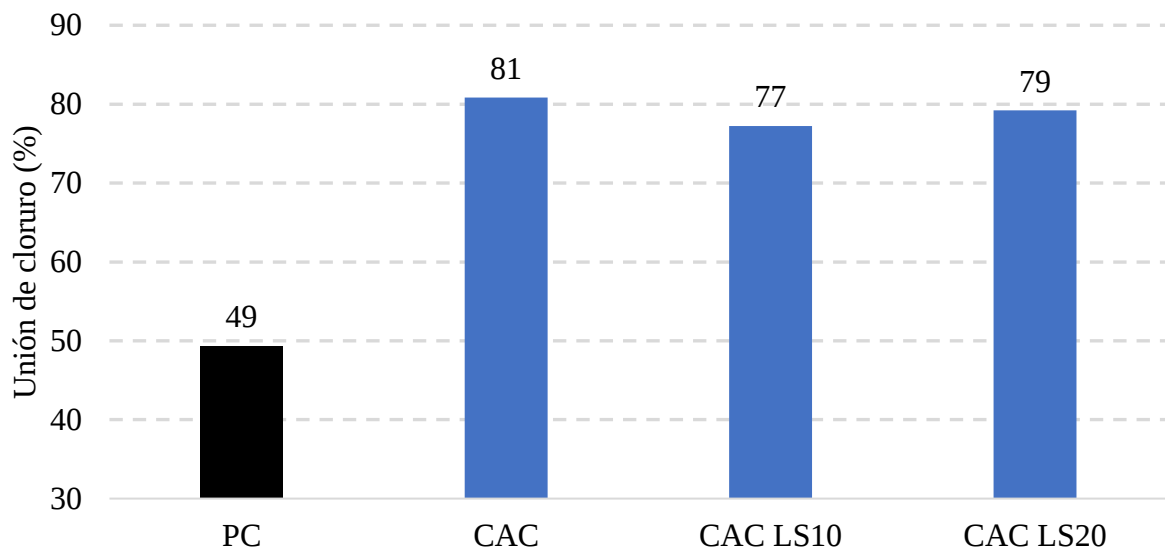
Figura 7. Combinación de cloruros para el sistema CAC (%)
