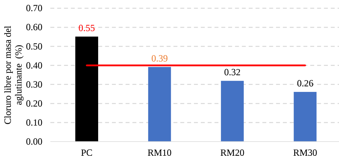
Figura 6. Porcentaje de cloruro libre por masa de ligante para el sistema de lodo rojo.
