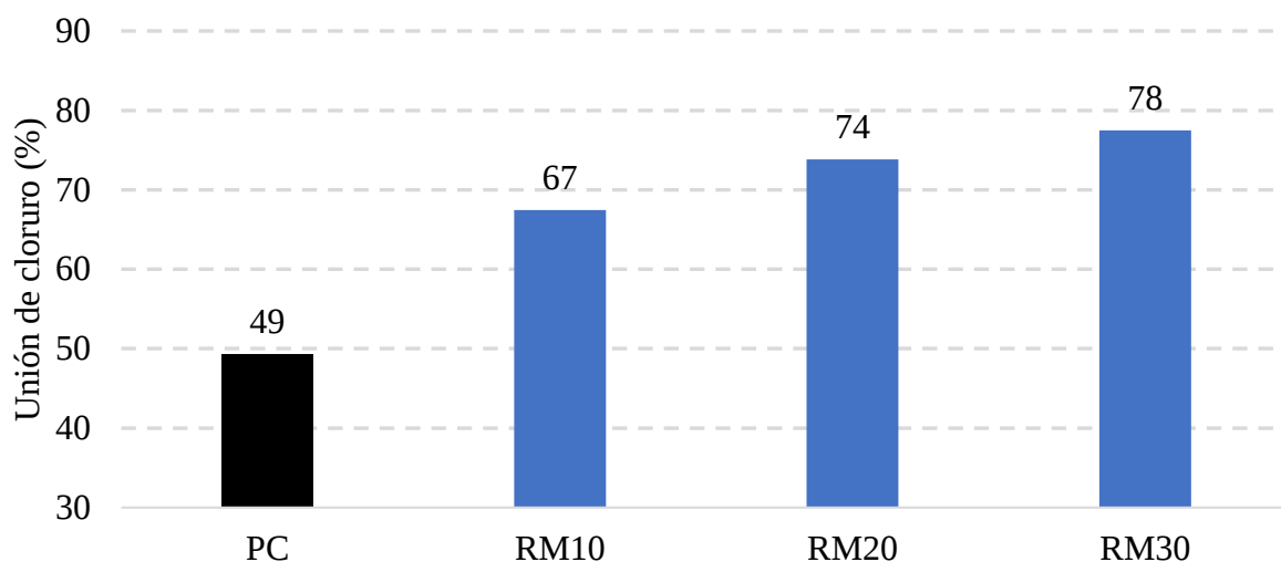
Figura 5. Vínculo de cloruro para el sistema de lodo rojo (%)
