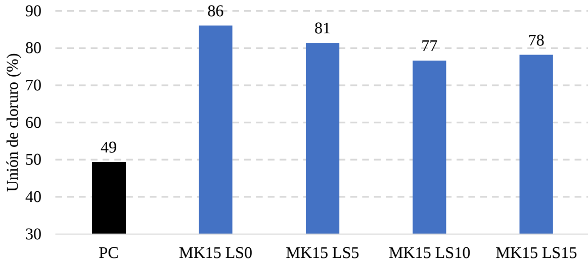
Figura 3. Enlace de cloruro para el sistema metacaolín-calcáreo, LS(%)
