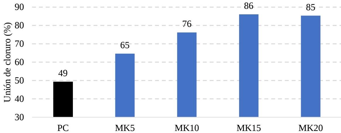
Figura 1. Vínculo de cloruro para el sistema de metacaolín, MK (%)
