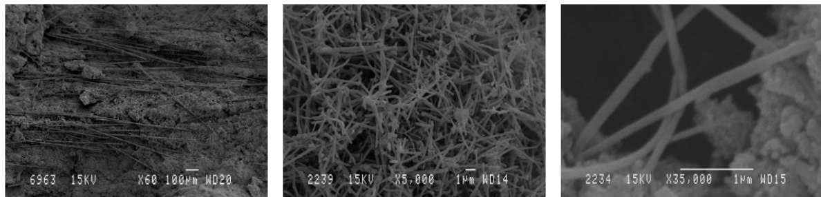
Figura 2. Imágenes de fibras de carbono (izquierda) y nanofibras de carbono (centro y derecha) embebidas en matrices cementicias.
